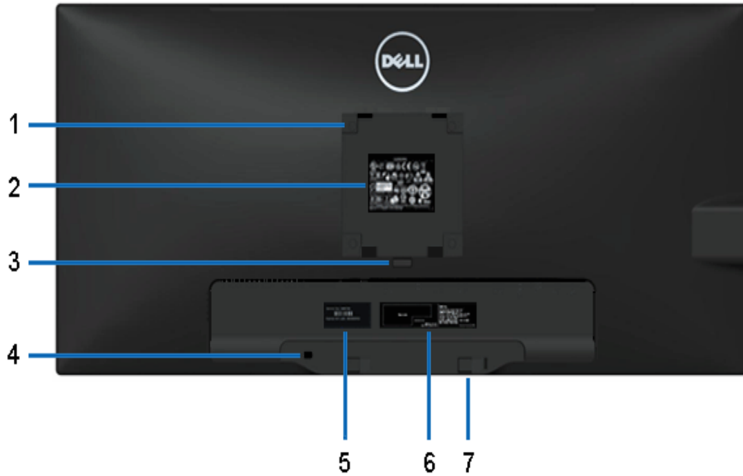
뒷면 모니터 스탠드가 장착된 상태의 뒷면
